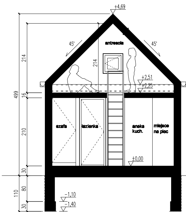
PRZEKRÓJ A-A
