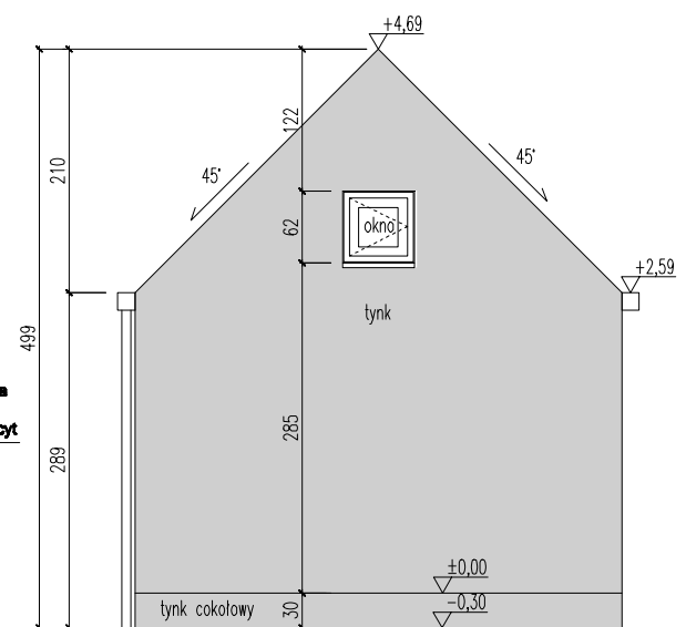
ELEWACJA C-D
