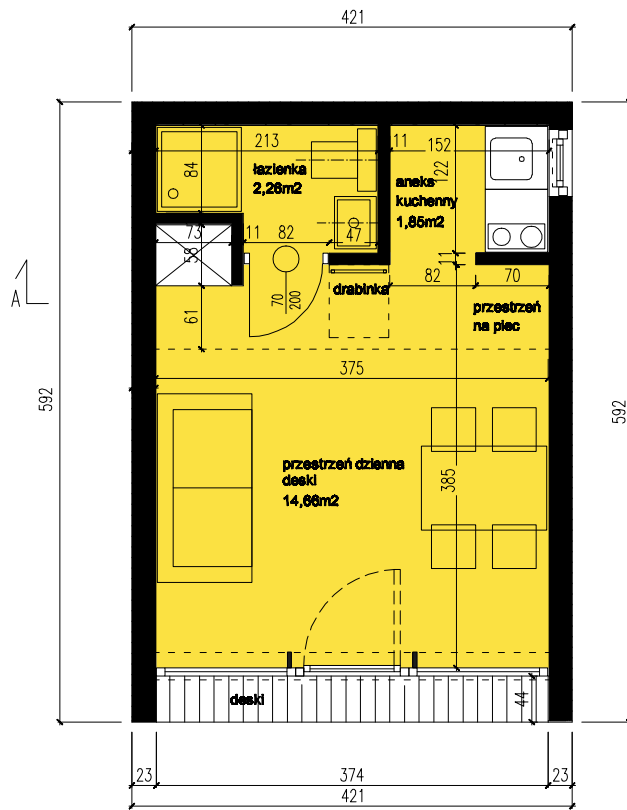
RZUT PARTERU
