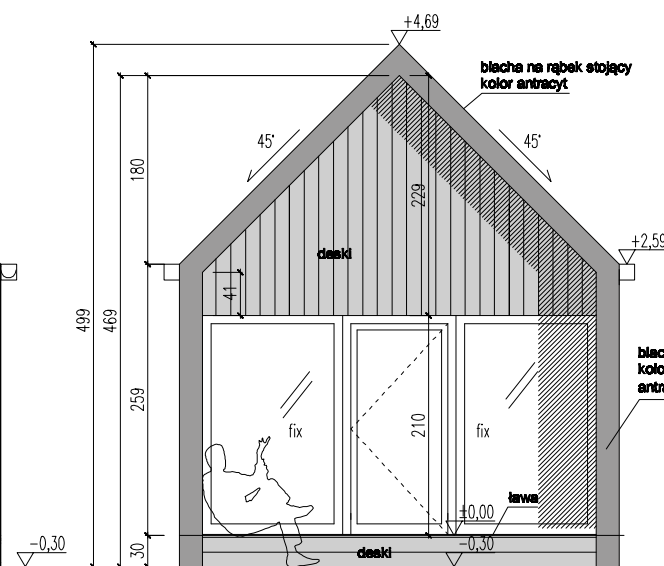
ELEWACJA A-B
